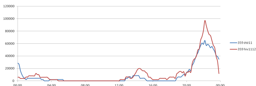
FIGURE 6.6 – Courbe de charges journalière (Puissance en fonction de l'heure) de la borne 359
