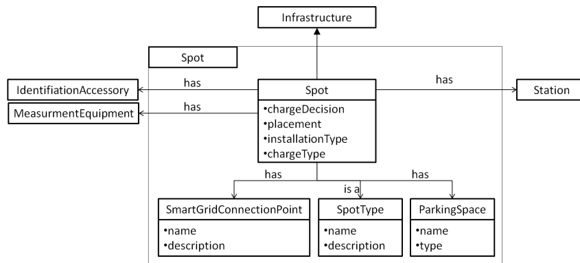
FIGURE 3.7 – Brigue de l'élément borne
